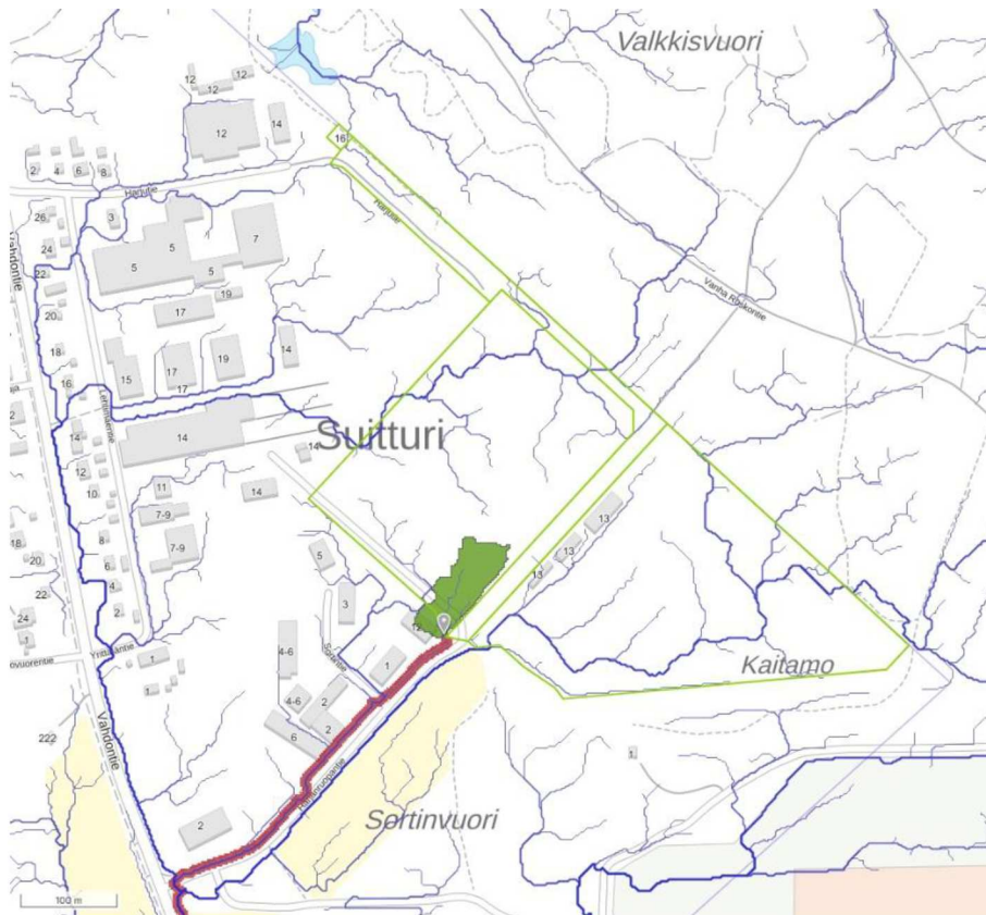
Kuva 16. Suunnittelualueen osavaluma-alue 3 (vihreä), jonka pinta-ala on 0,5 ha. Käyttötarkoitusalueiden rajat merkitty vaalean vihreällä ja vesien poistvirtausreitti punaisella. (Scalگو Live)
