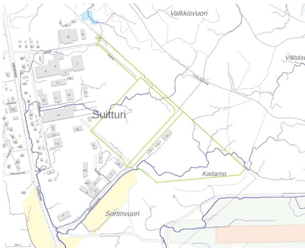
Kuva 11. Suunnittelualueen virtausreitit, joiden yläpuolinen valuma-alue on yli 0,5 ha. Käytötarkoitusalueiden rajat merkitty vihreällä. (Scalgo Live)
