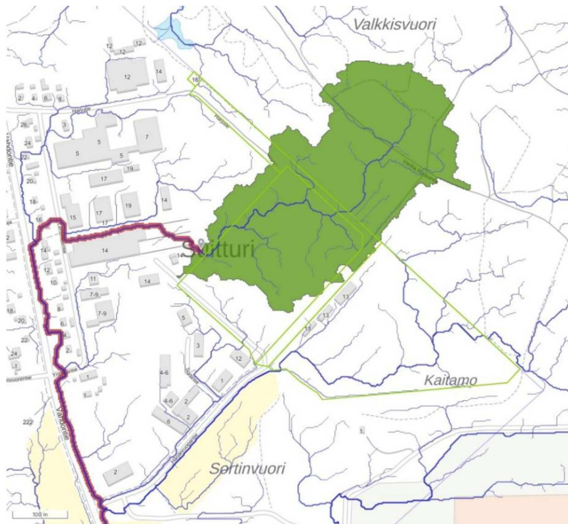
Kuva 14. Suunnittelualueen osavalmu-alue 1 (vihreä), jonka pinta-ala on 0,12 km 2 . Käyttötarkoituksalueiden rajat merkitty vaalean vihreällä ja vesien poisvirtaamisreitti punaisella. (Scalgo Live)
