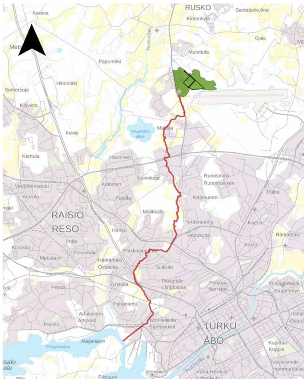
Kuva 13. Suunnittelualan hulevesien virtausreitti (Scalgo Live). Virtausreitti merkitty punaisella, suunnittelualue mustalla rajauksella ja valuma-alue vihreällä.
