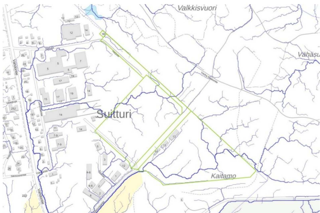
Kuva 12. Suunnittelualueen virtausreitit, joiden yläpuolinen valuma-alue on yli 0,1 ha. Käytötarkoitusalueiden rajat merkitty vihreällä. (Scalgo Live)
