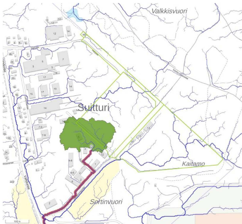
Kuva 15. Suunnittelualueen osavalmu-alue 2 (vihreä), jonka pinta-ala on 2,7 ha. Käyttötarkoituksalueiden rajat merkitty vaalean vihreällä ja vesien poisvirtaamisreitti punaisella. (Scalgo Live)
