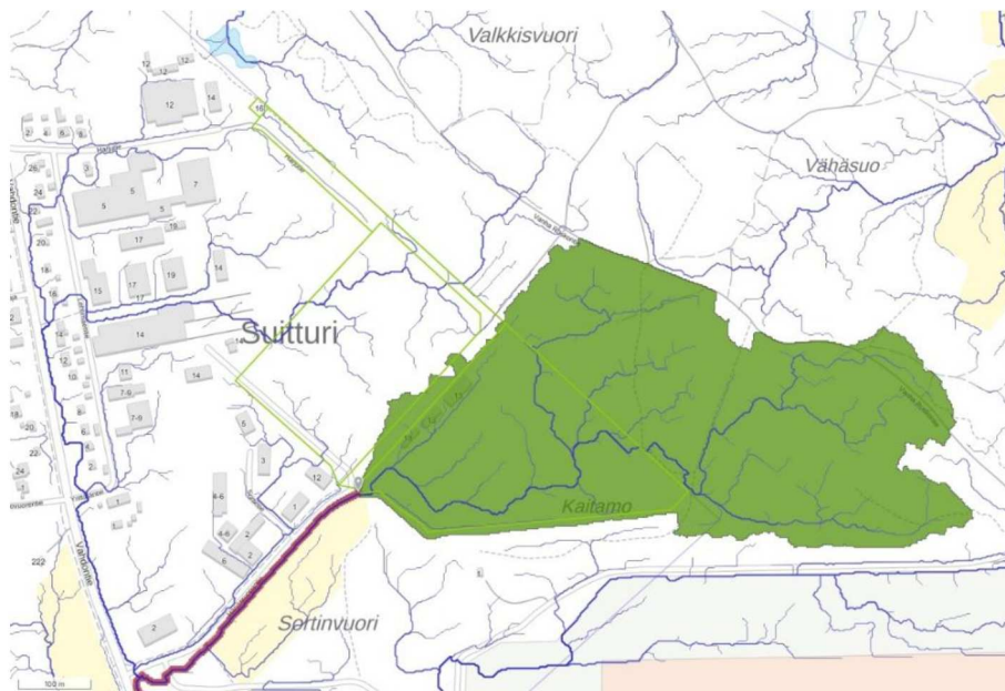
Kuva 17. Suunnittelualueen osavaluma-alue 4 (vihreä), jonka pinta-ala on 0,23 km 2 . Käyttötarkoitusalueiden rajat merkitty vaalean vihreällä ja vesien poistvirtausreitti punaisella. (Scalگو Live)
